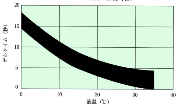
サンコーボールSW3A-S1 [参考図]
