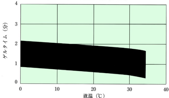
サンコーボールSW3A-M1 [参考図]
