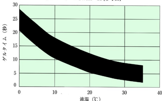
サンコーボールSW3A-S2 [参考図]
