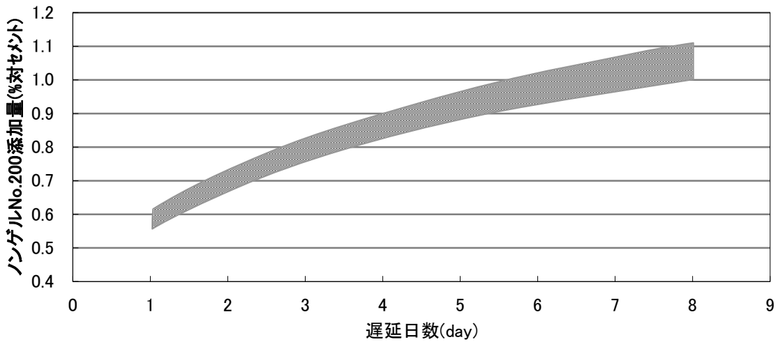
サンコーノンゲルNo.200添加量と遅延日数
