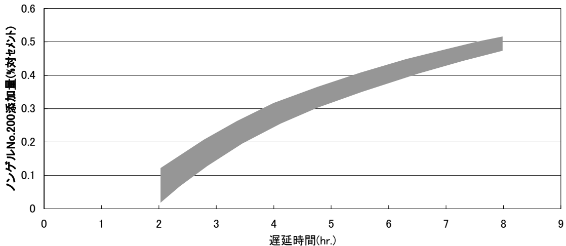
サンコーノンゲルNo.200添加量と遅延時間
