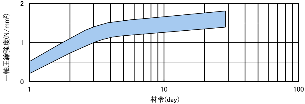
一軸圧縮強度 (20°C 湿潤養生)
