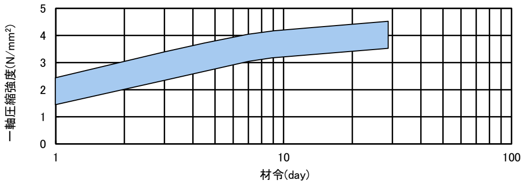
一軸圧縮強度 (20°C 湿潤養生)
