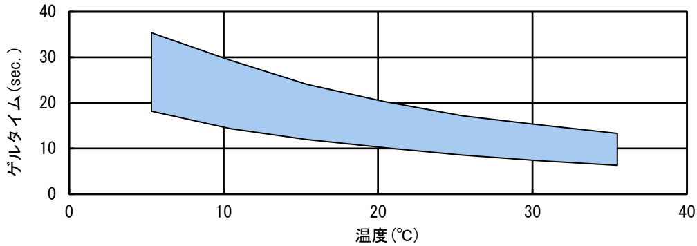
液温とゲルタイムの関係
