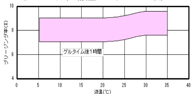
ブリージング率 (液温 20℃ : 7~8%)
