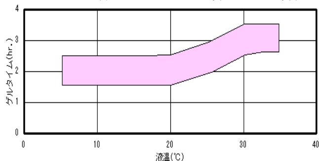
ゲルタイム (液温 20℃ : 90分~150分)
