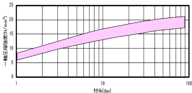
一軸圧縮強度(28日後 : 約 17 (N/mm 2 ))
